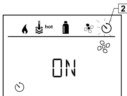
Afb. 132: Indicatie tijdschakelklok
