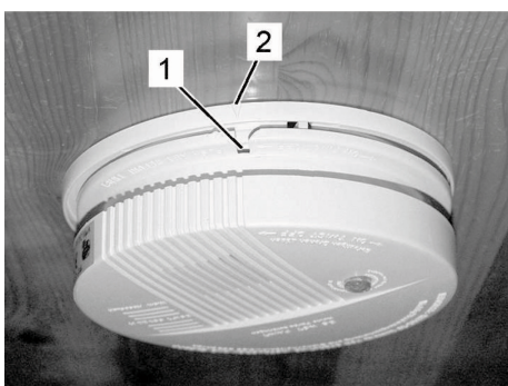
Afb. 207: Behuizing plaatsen
