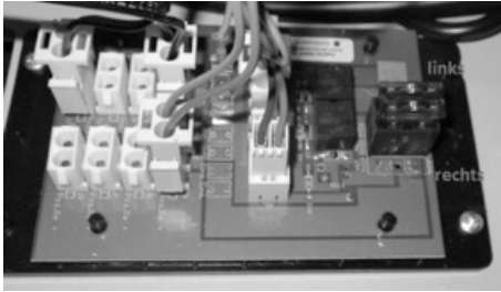
Afb. 6: Interface-module
