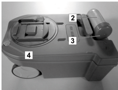
Afb. 183: Fecaliëntank legen
