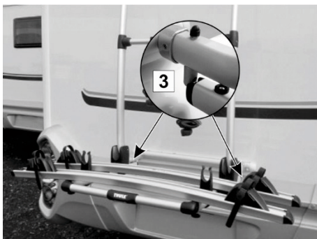
Afb. 23: Arrêteerinrichtingen vergrendelen
