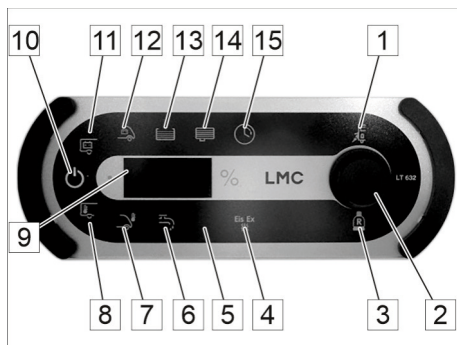
Afb. 58: Bedienings- en controlepaneel LT 632
