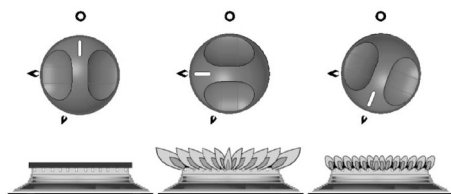
Afb. 186: Standen van de bedieningselementen: UIT, grote vlam, kleine vlam
