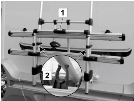
Afb. 22: Fietsendrager opklappen
