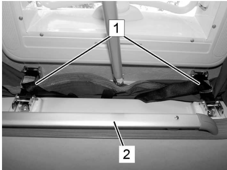
Afb. 173: Hefdak uitklappen
