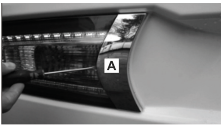
Afb. 201: Achterlicht
