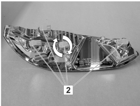
Afb. 203: Achterlicht (achterzijde)
