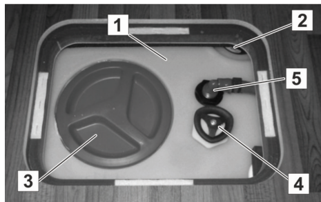
Afb. 78: Plaatsing onder de vloer
