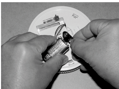
Afb. 152: Blokbatteij vervangen
