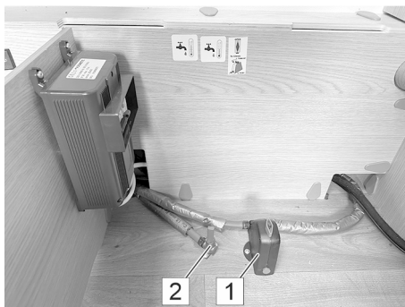
Afb. 73: Aftapkranen
