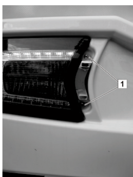
Afb. 148: Achterlicht afnemen
