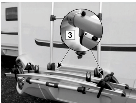
Afb. 24: Arrêteerinrichtingen vergrendelen
