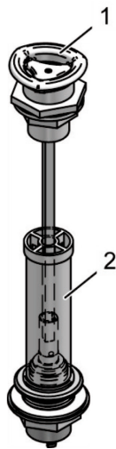
Afb. 79: Combi-aftapkraan
