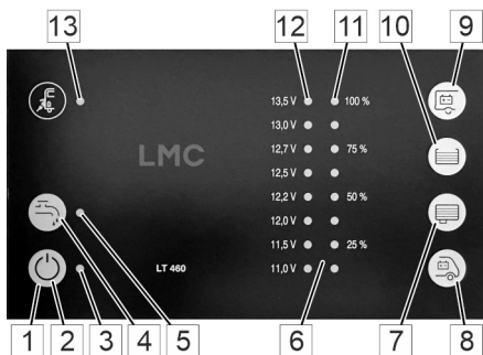
Afb. 52: Bedienings- en controlepaneel LT 460 A
