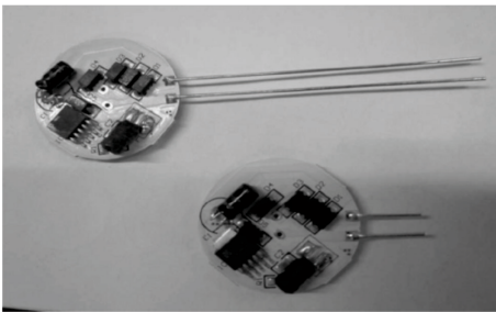
Afb. 142: Contacten inkorten
