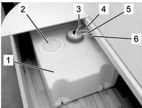
Afb. 89: verswatertank, voorbeeld
