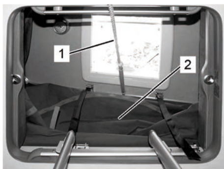
Afb. 187 trekkoord (1), vouwbalg (2)
