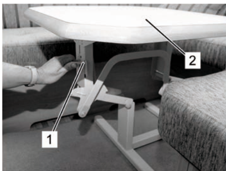
Afb. 173: tafel met heftafeldraagconstructie
