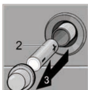
Afb. 214: Batterijvervanging bij batterijontsteker (alleen wanneer aanwezig)
