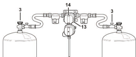
Afb. 110: Gasdrukregelset
