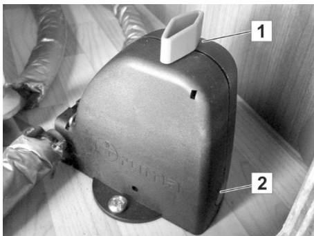
Afb. 105: Veiligheidsaftapkraan gesloten
