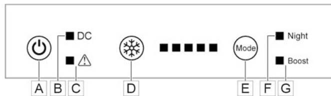
Afb. 216: Bedieningselementen 12 V compressor-koelkast
