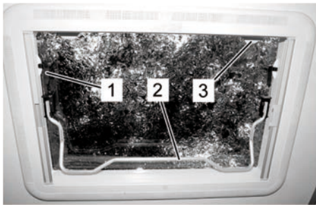
Afb. 122: Hef-kanteldak Heki 2 bedienen
