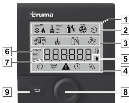
Afb. 133: Digitaal TRUMA-bedieningspaneel CP plus
