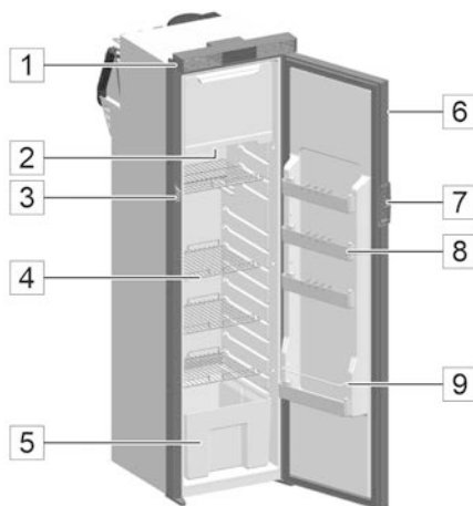
Afb. 215: 12 V compressor-koelkast
