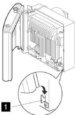
Afb. 127: bekleding van verwarming opgedraaid
