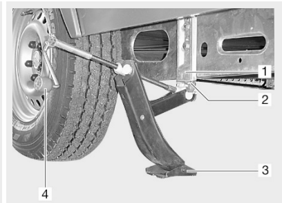
Afb. 221: Wagenkrik, AL-KO
