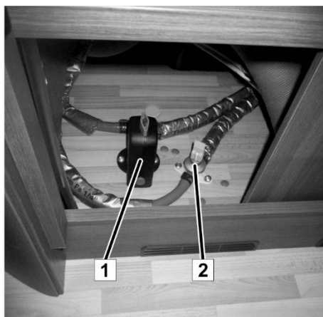
Afb. 103: Aftapkranen TRUMA combi verwarming
