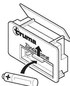
Afb. 128: batterijvervangning
