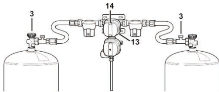
Afb. 113: Gasdrukregelset
